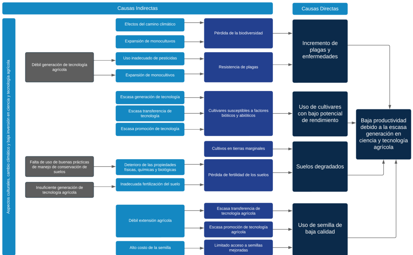
Figura 2. Modelo conceptual
