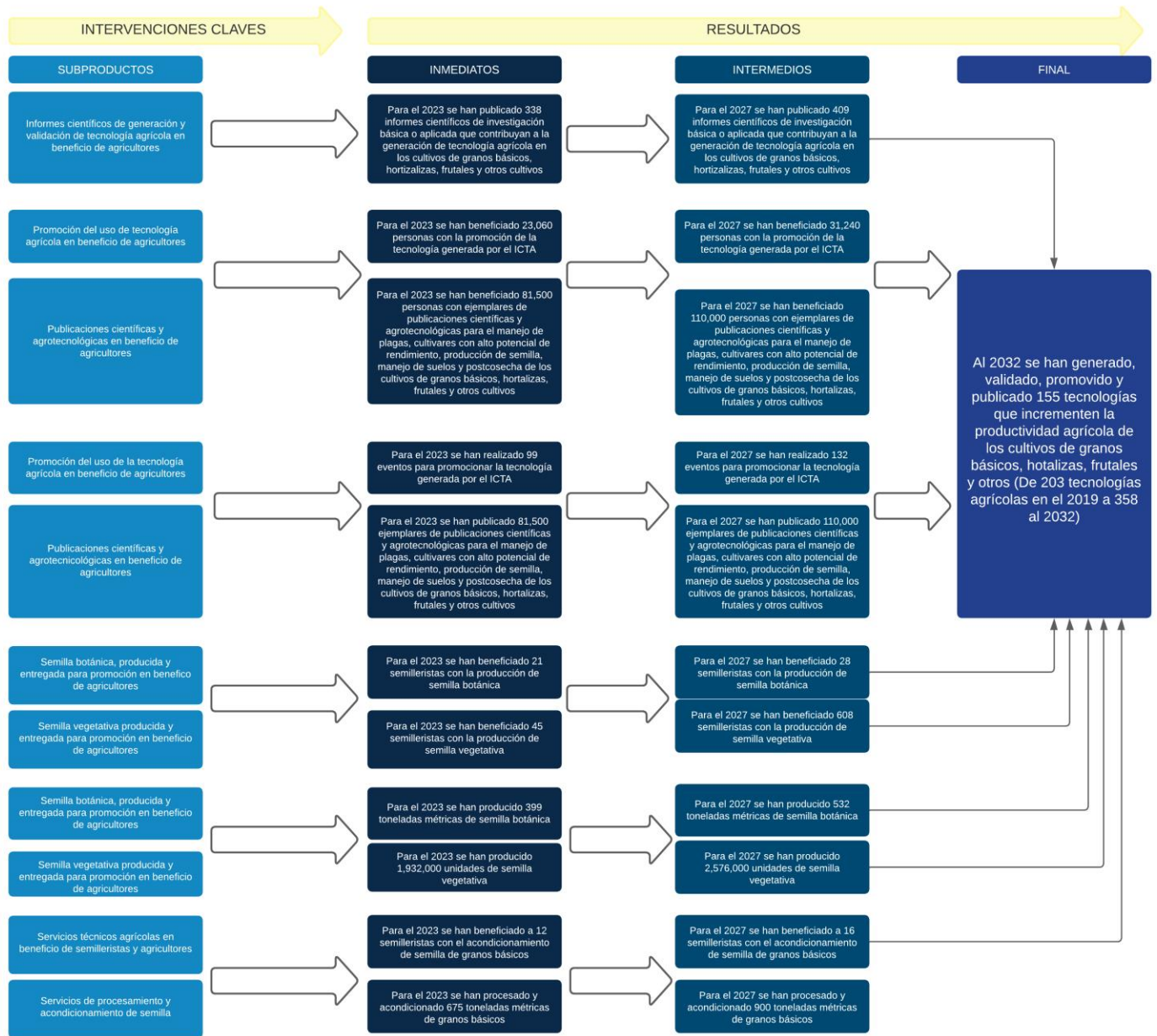
Figura 9. Modelo lógico
