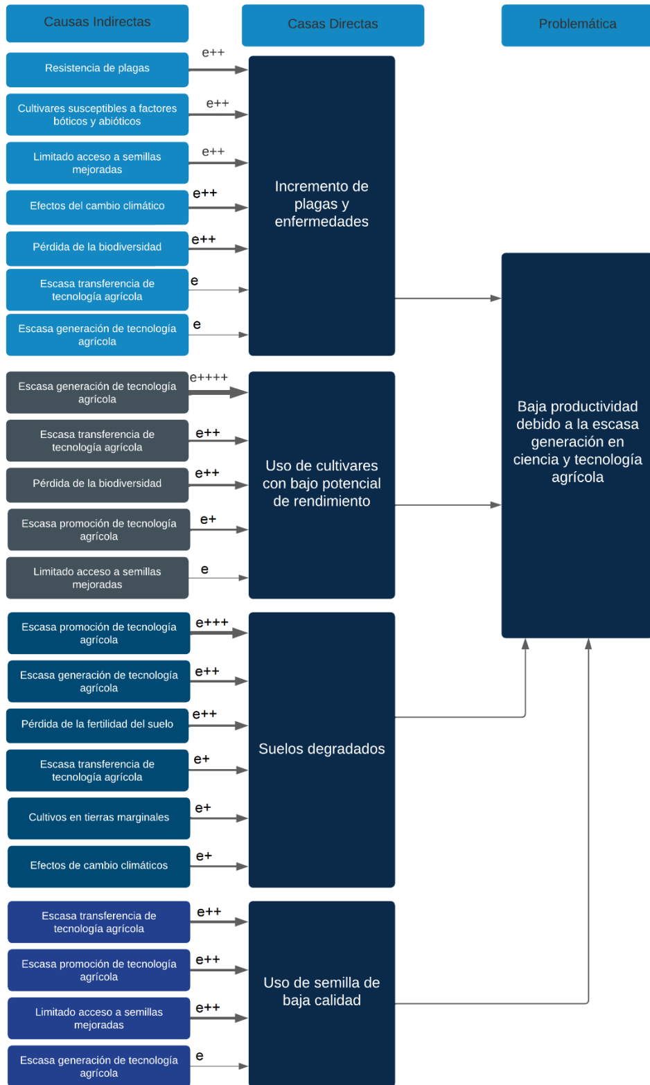
Figura 3. Modelo explicativo
